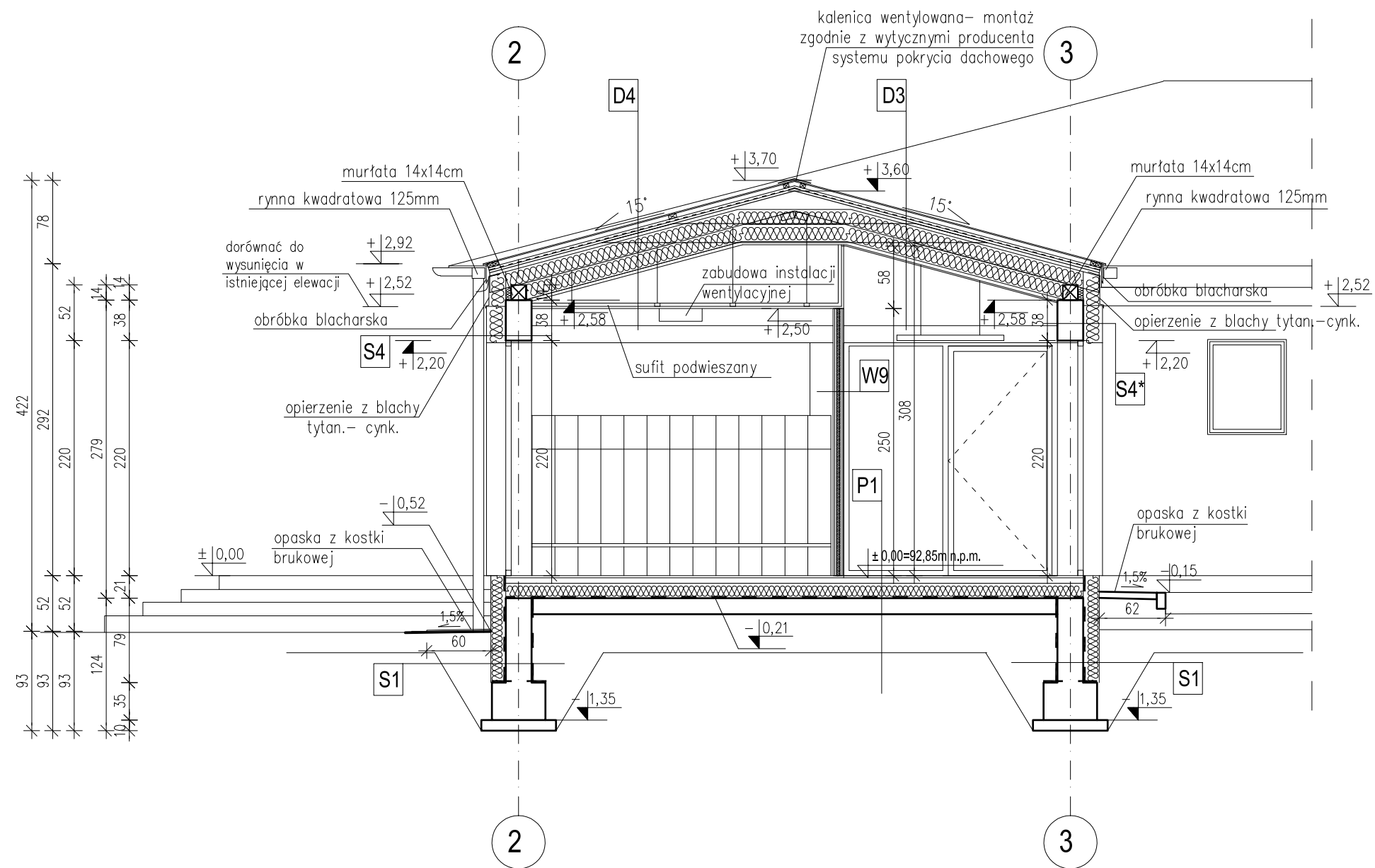
Przekrój A-A
