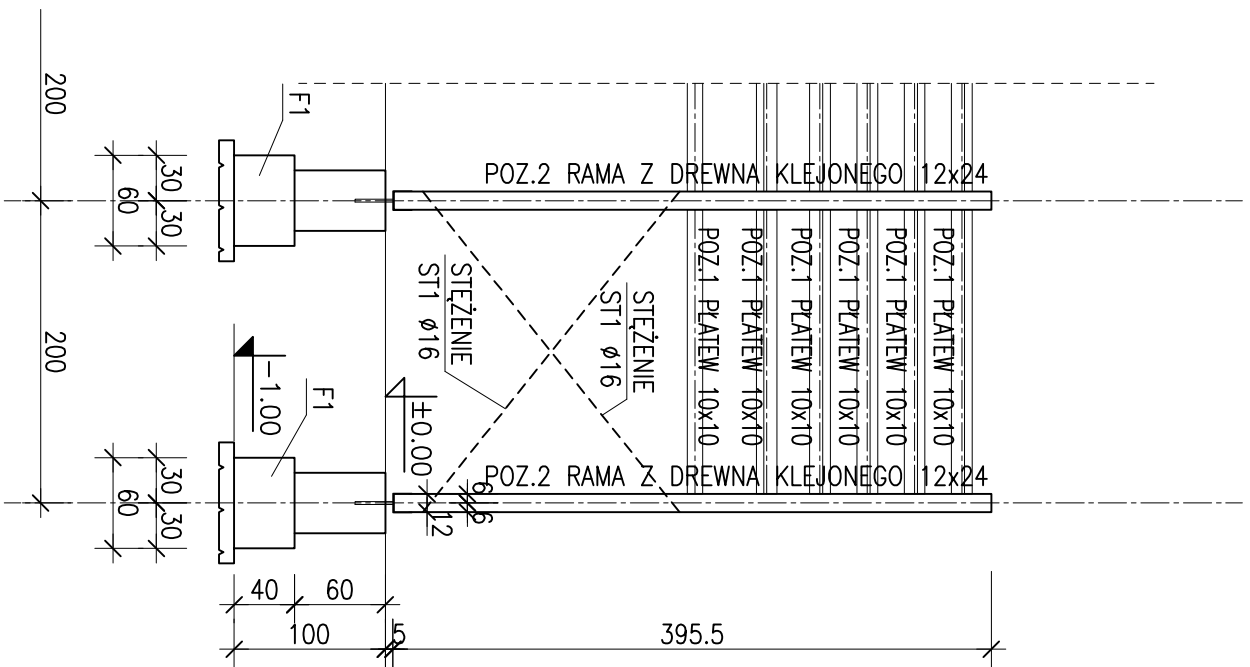
WIDOK SKRAJNEGO POLA ZE STEZENIEM PIONOWYM 1:50
