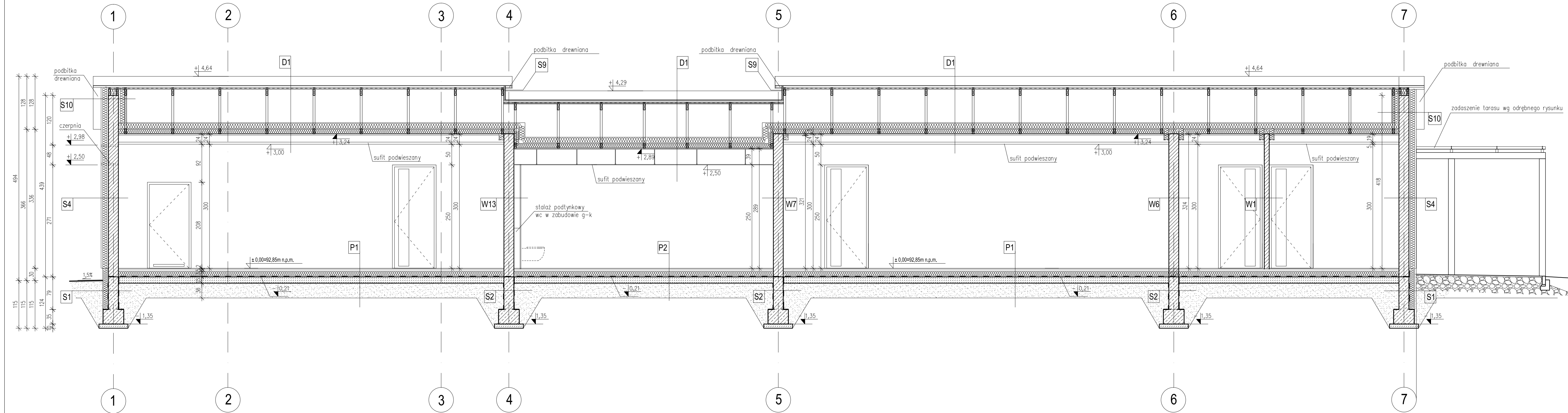
Przekrój C-C
