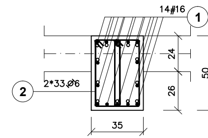
PRZEKRÓJ 1-1
