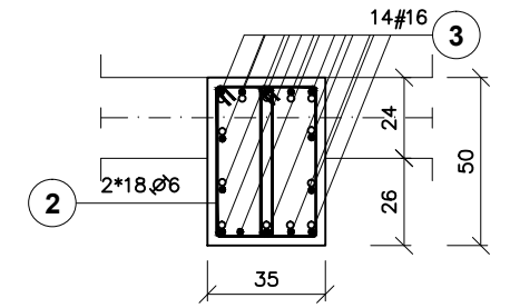
PRZEKRÓJ 2-2
