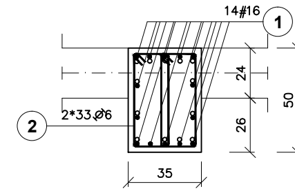
PRZEKRÓJ 1-1
