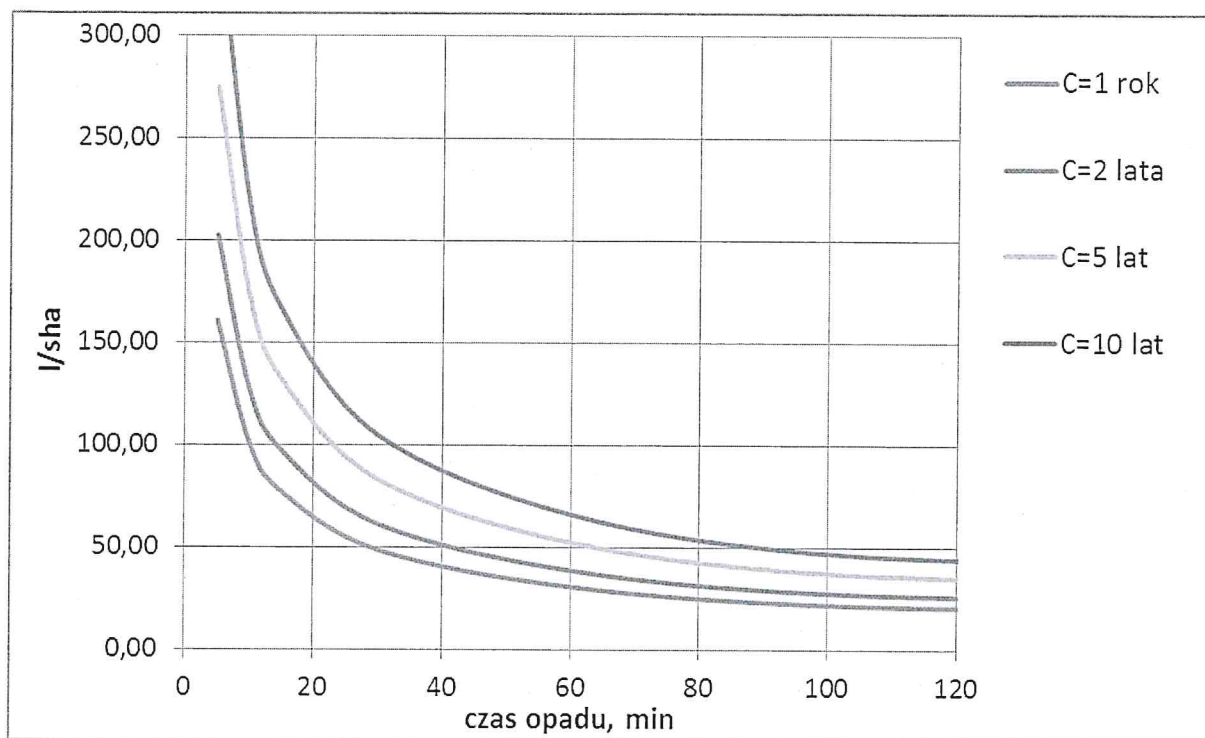
Rysunek 2. Opad miarodajny – zależność między czasem trwania a natężeniem opadu
