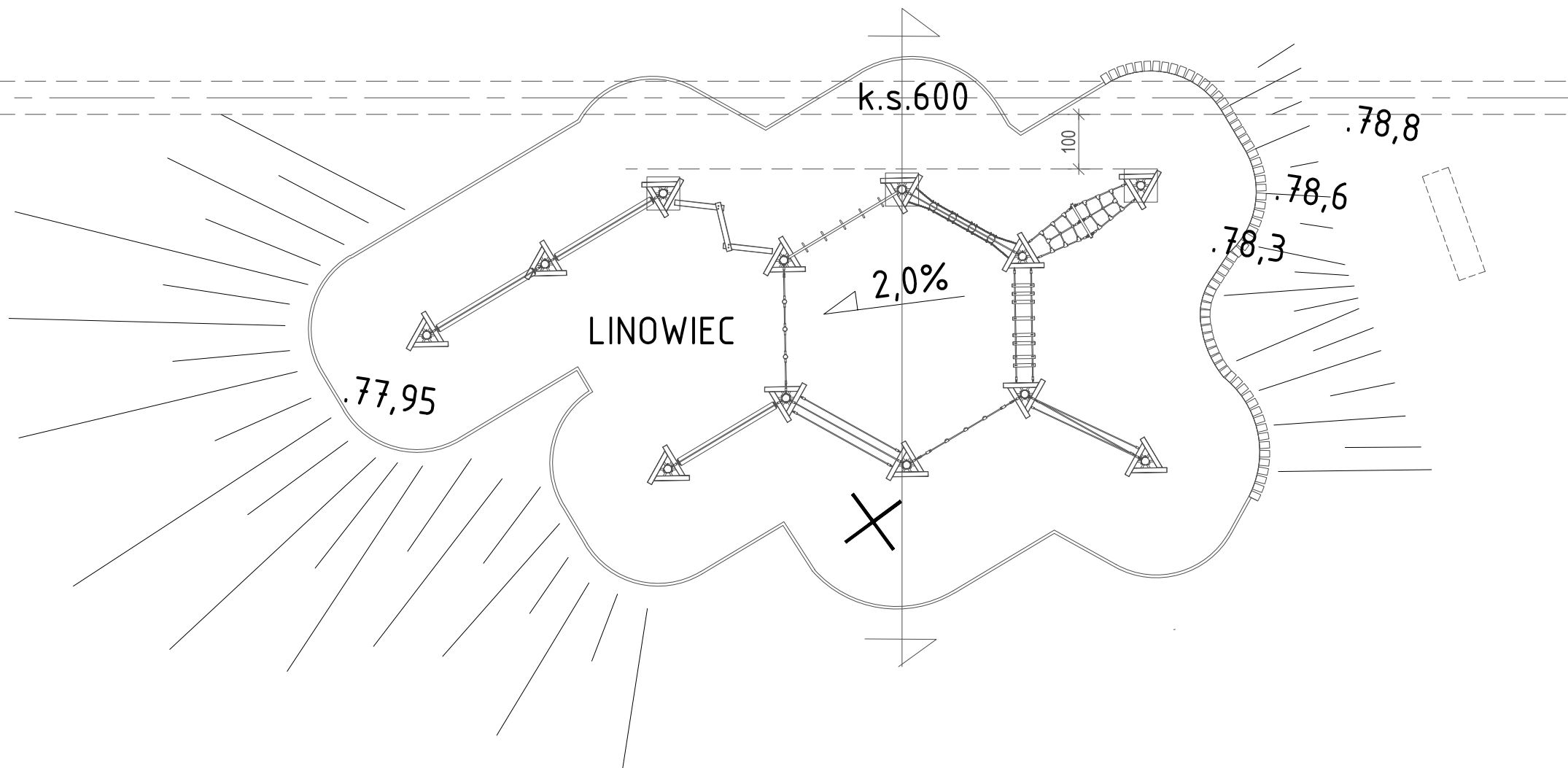
RZUT URZĄDZENIA LINOWEGO ZBLIŻENIE DO SIECI K.S.600
