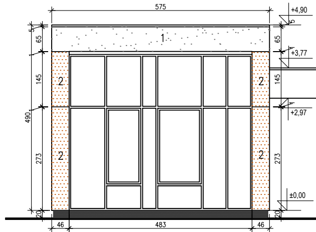
ELEWACJA E7-E7
