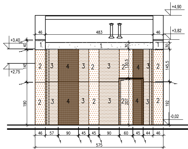
ELEWACJA E8-E8
