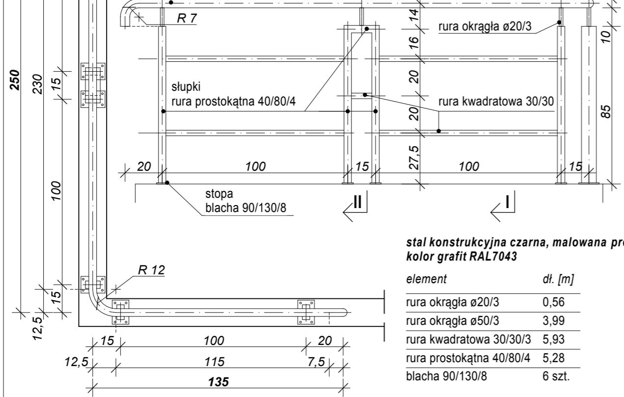
BALUSTRADA 1 ZESTAWIENIE ELEMENTÓW
