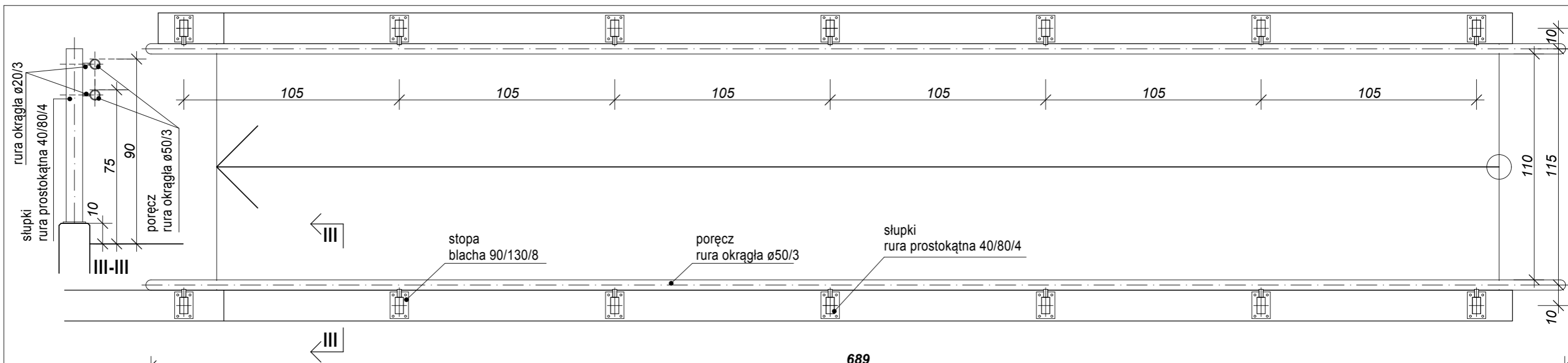
BALUSTRADA 2 ZESTAWIENIE ELEMENTÓW
