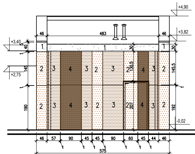
ELEWACJA E8-E8
