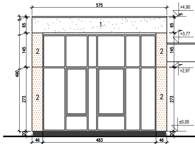
ELEWACJA E7-E7
