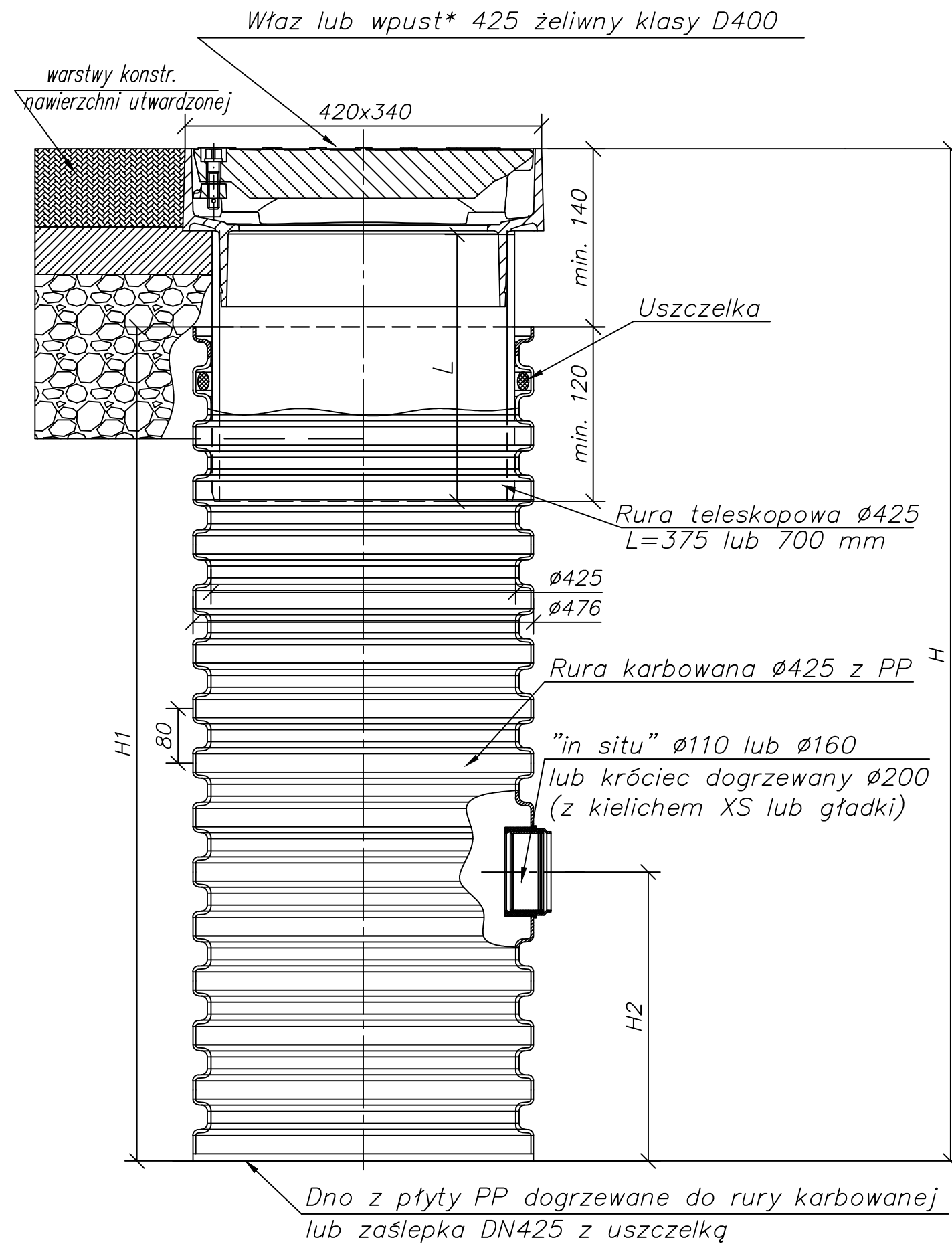
Studzienka osadnikowa ø425 z rurą teleskopową
