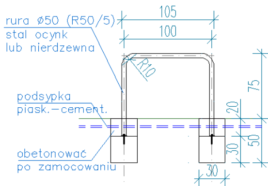
Rysunek 3. Przekrój przez stojak
