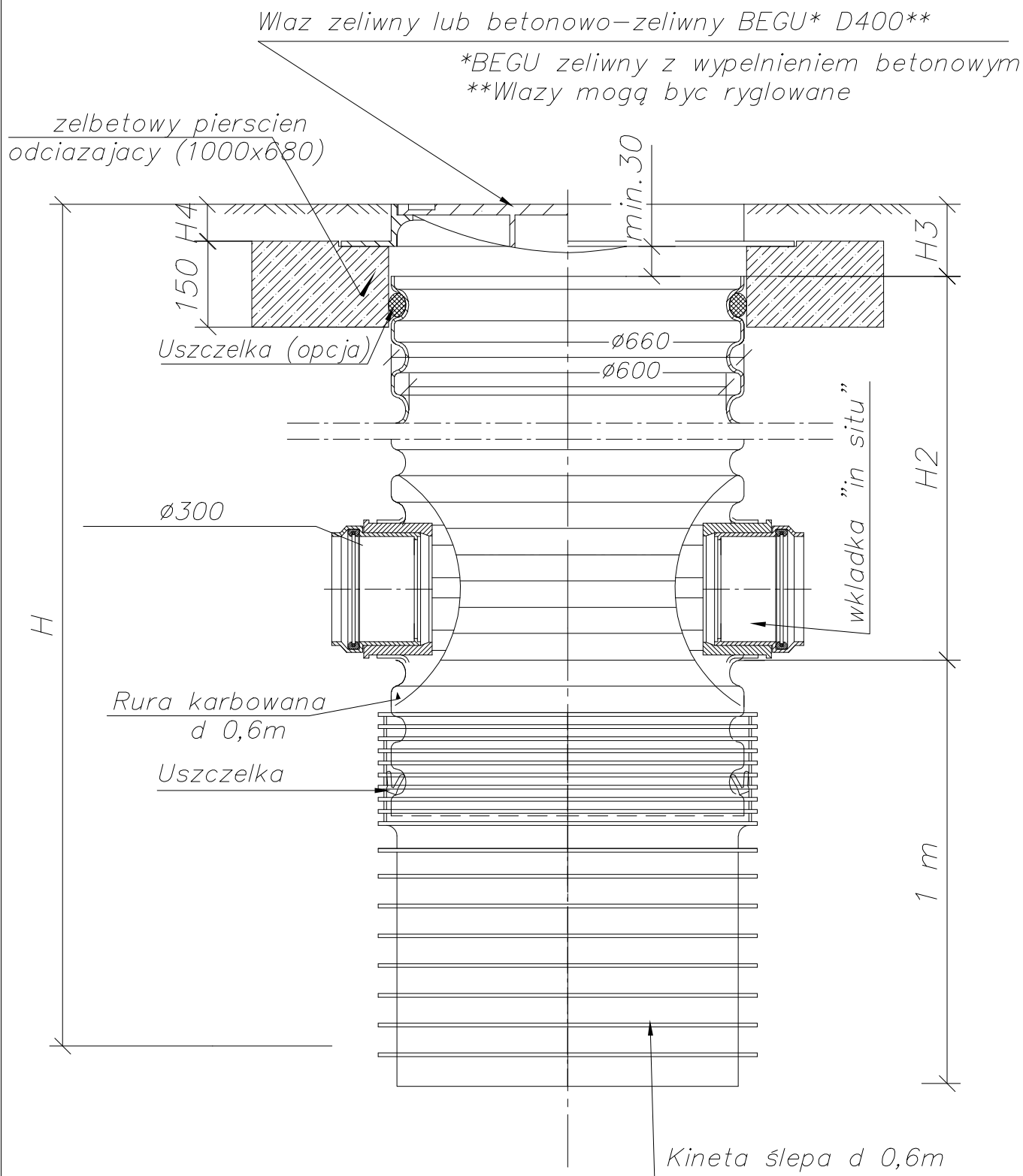
Studzienka ślepa d 0,6m z złbetowym pierścieniem odciążającym oraz włazem klasy D400
