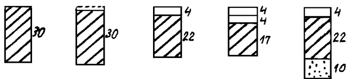
Rys. 4. Przykładowe wybrane konstrukcje nawierzchni utwardzonego pobocza z kruszywa łamanego niezwiązane
