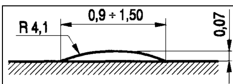
Rys. 5. Przekrój poprzeczny progów zwalniającego liniowego o zmniejszonej szerokości (progów skróconego) w przekroju poprzecznym jezdni
