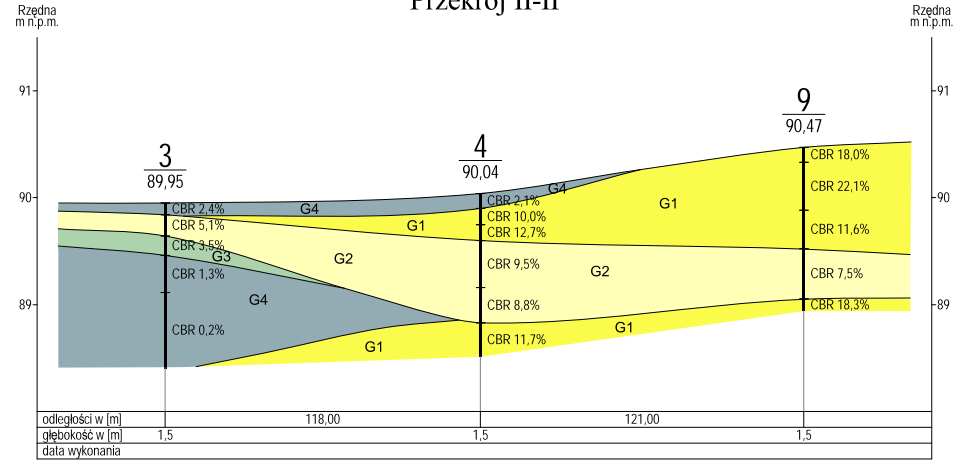
Przekrój II-II
