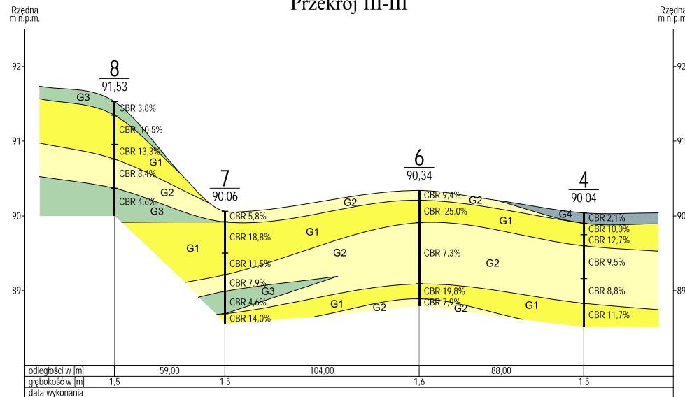
Przekrój III-III
