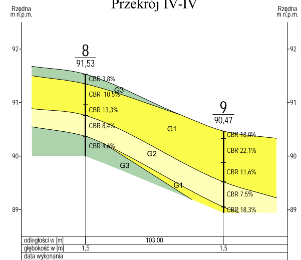
Przekrój IV-IV
