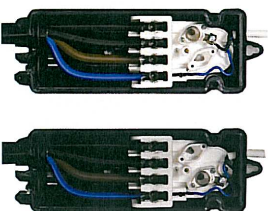
Możliwość przekazania gniazda bezpiecznikowego w złączu TB-1
