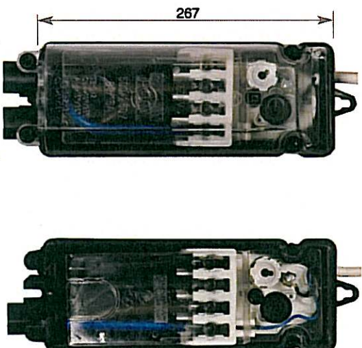
złącza słupowe typu TB-1 (widok z pokrywą pośrodkną)
