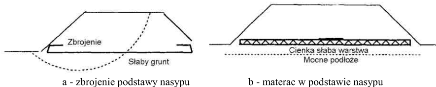
Rys. 2.2. Przykłady zbrojenia nasypów geosyntezykami
