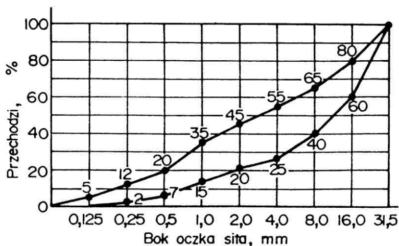
Rysunek 1. Graniczne krzywe uziarnienia do betonu B 7,5 od 0 do 31,5 mm.
