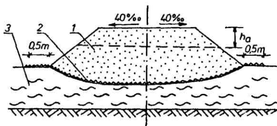
Rys. 2.1. Schemat nasypu na gruncie słabonośnym z zastosowaniem geosyntezyki
