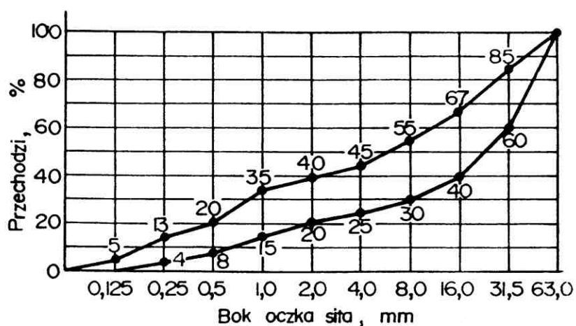
Rysunek 2. Graniczne krzywe uziarnienia kruszywa do betonu B 7,5 od 0 do 63 mm.
