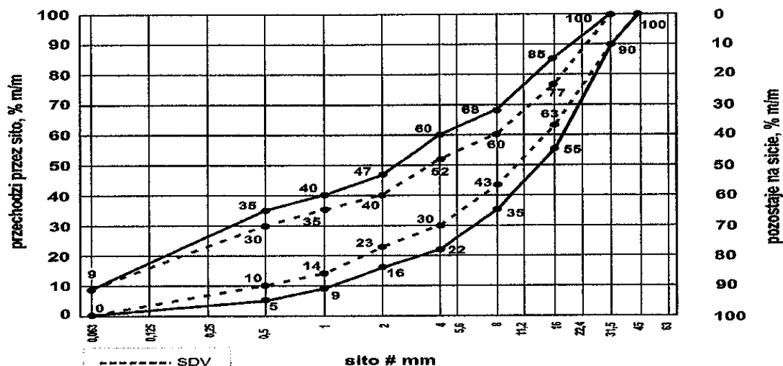
Rysunek 1. Krzywa uziarnienia dla podbudowy
