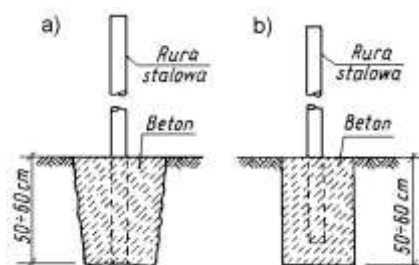
Rys. 4. Przykład ustawiania słupków ogrodzenia (wg [6])
