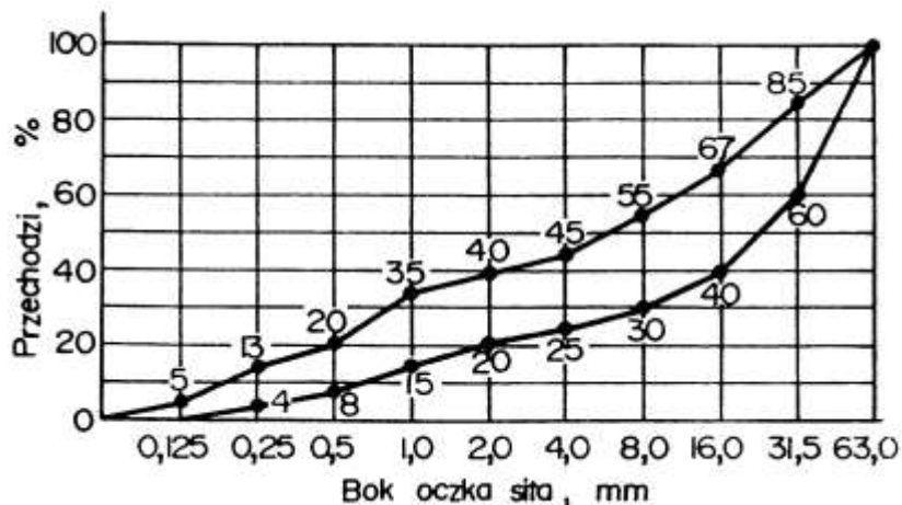
Rysunek 2. Graniczne krzywe uziarnienia kruszywa do betonu B 7,5 od 0 do 63 mm.
