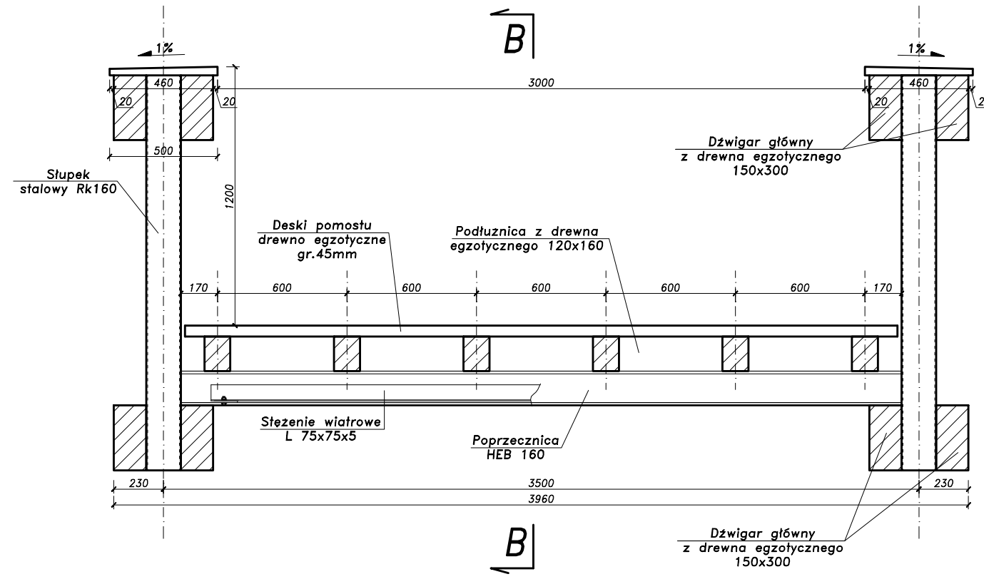
Przekrój poprzeczny A-A skala 1:25
