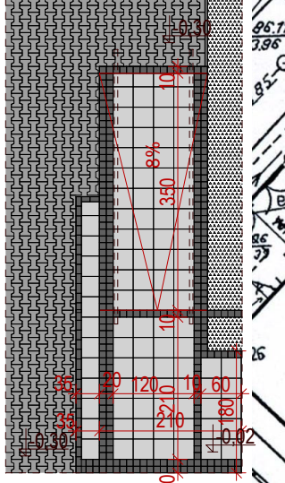
D04 - detal -skala 1:100
