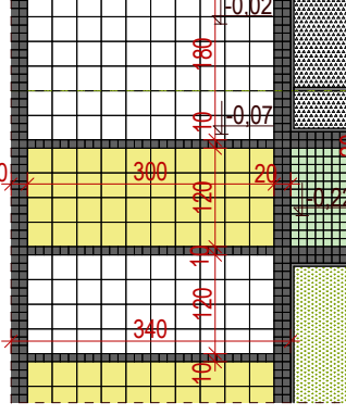
D02 - detal w skali 1:100
