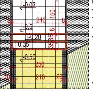
D03 - detal w skali 1:100
