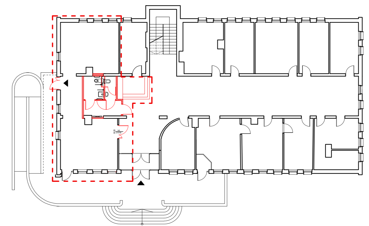
rzut parteru - schemat skala 1:200
