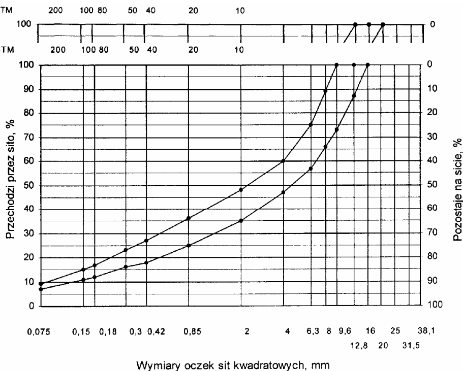
Rys. 1. Krzywe graniczne uziarnienia mieszanki mineralnej BA od 0 do 16 mm do warstwy ścieralnej nawierzchni drogi
