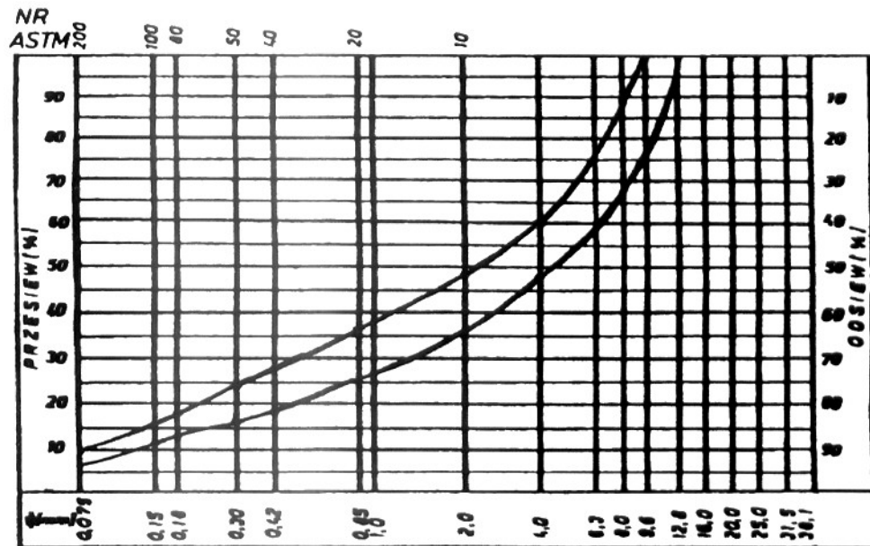
Rys. nr 2. Krzywe graniczne uziarnienia mieszanki mineralnej 0 ÷ 12,8 mm do warstwy ścieralnej z betonu asfaltowego
