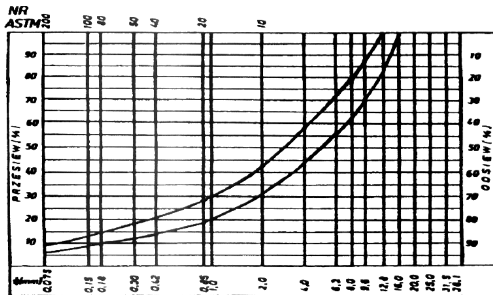
Rys. nr 1. Krzywe graniczne uziarnienia mieszanki mineralnej 0 ÷ 16 mm do warstwy ścieralnej z betonu asfaltowego
