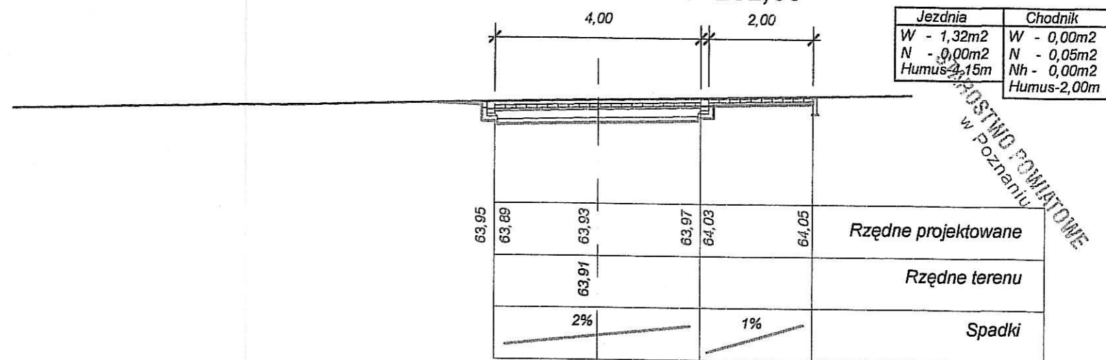
KM 0+282,00
