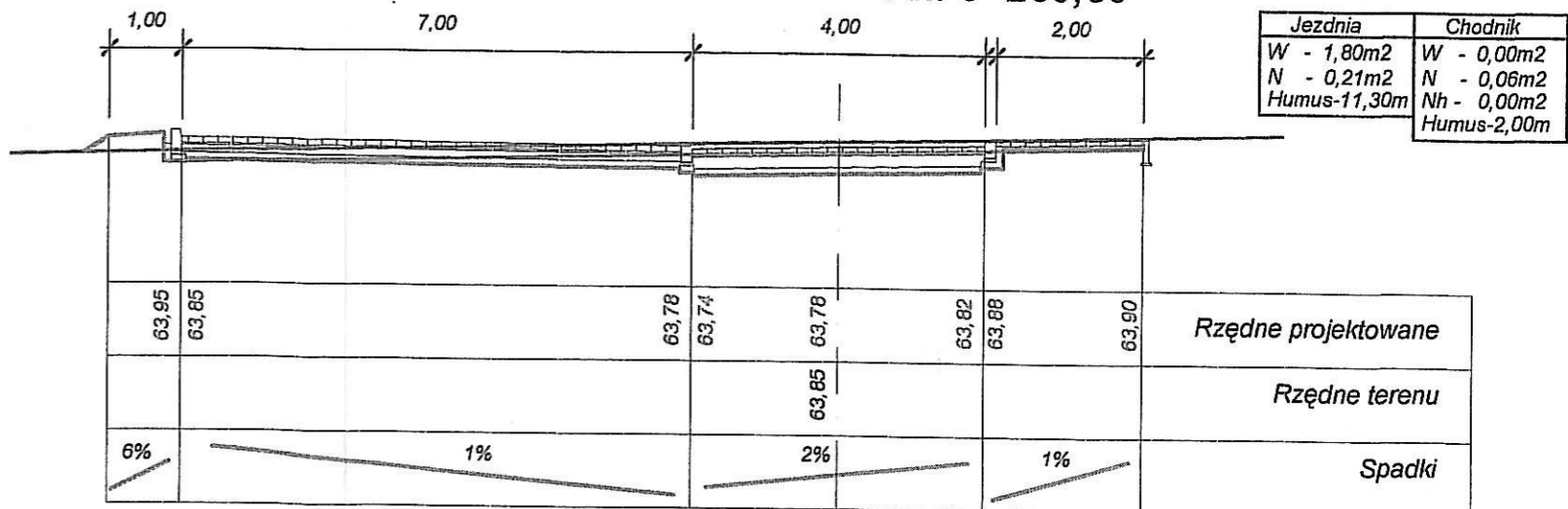
KM 0+269,50
